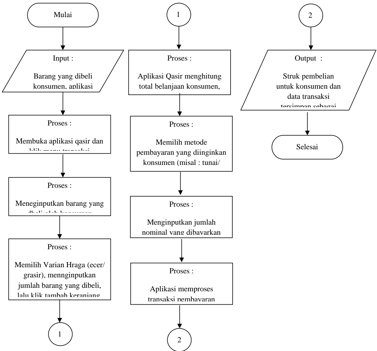
Gambar 12 Flowchart Sistem Informasi Akuntansi Penerimaan Kas Dengan Menerapkan Aplikasi Qasir
