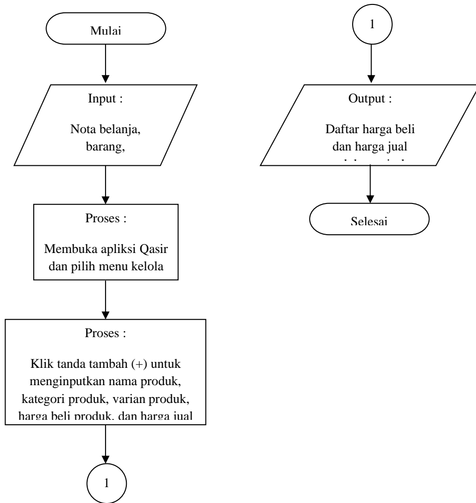
Gambar 4 Flowchart Sistem Informasi Akuntansi Pencatatan Daftar Harga Barang Dagang Dengan Menerapkan Aplikasi Qasir
