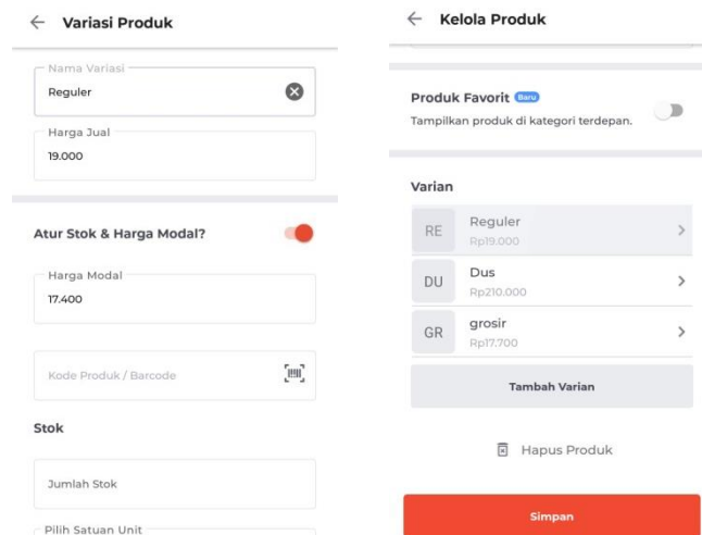
Gambar 6 Tampilan Menu Penginputan Harga Produk pada Aplikasi Qasir
