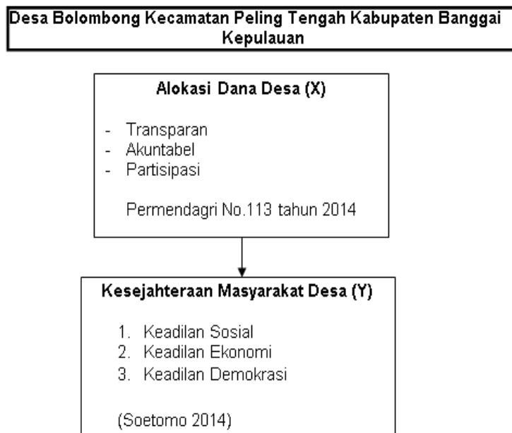
Gambar 1 Kerangka Pemikiran
